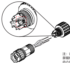
图 4.18 连接电缆线
